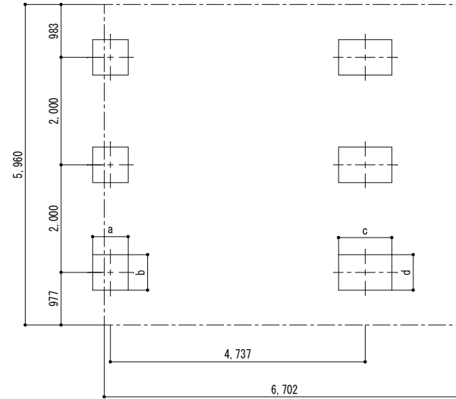
■ 基礎配置図
